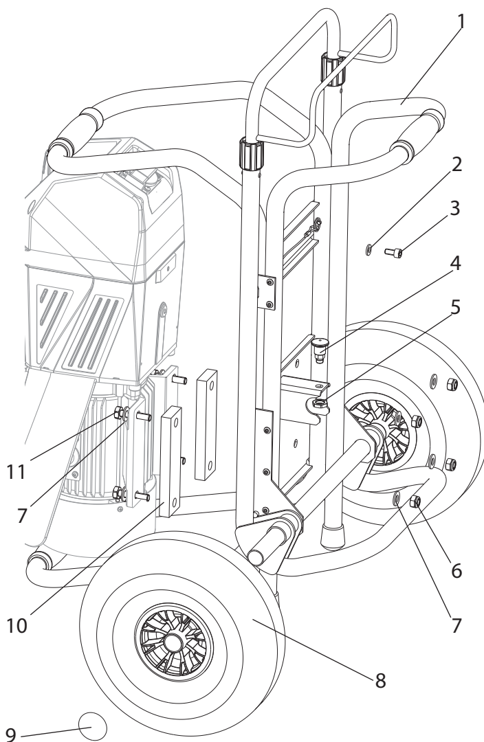
Ersatzteilbild Wagen
