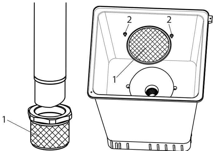
starres Ansaugrohr
